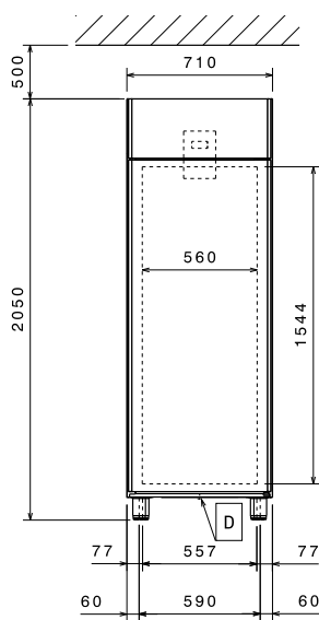
Front aanzicht
